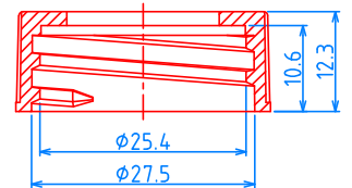
(28/400) CAP, P=1"x8 TPI
