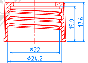
(24/415) CAP, P=1"x8 TPI
