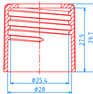
(30/400) CAP, P=1"x8 TPI
