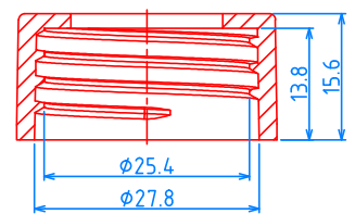
(28/400) CAP, P=1"x8 TPI
