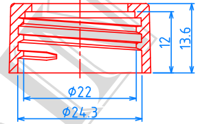
(24/410) CAP, P=1"x8 TPI
