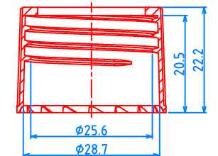
(30/400) CAP, P=1"x8 TPI
