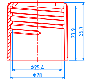
(28/420) CAP, P=1"x8 TPI
