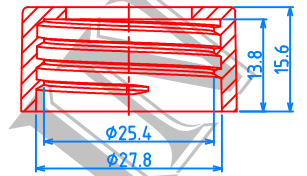
(28/400) CAP, P=1"x8 TPI
