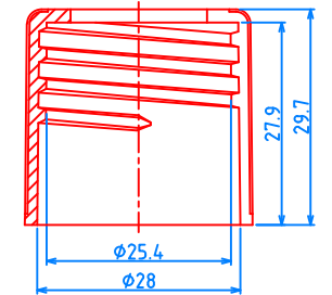
(28/415) CAP, P=1"x8 TPI
