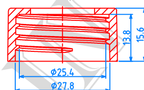
(28/400) CAP, P=1"x8 TPI
