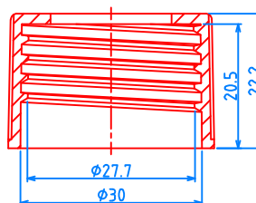
(30/400) CAP, P=1"x8 TPI
