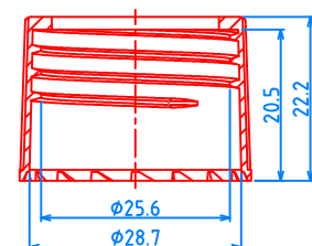
(28/420) CAP, P=1"x8 TPI
