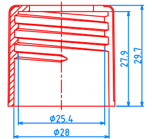
(28/420) CAP, P=1"x8 TPI
