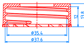
(38/400) (中) CAP, P=1"x8 TPI
