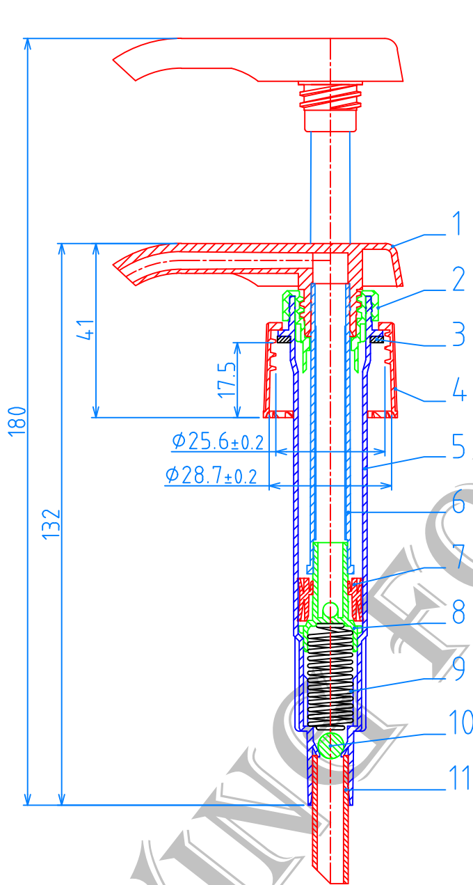
(38/400) CAP, P=1"x6 TPI (中)
