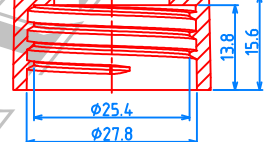
(28/400) CAP, P=1"x8 TPI
