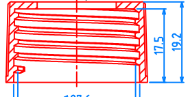
(30/400) CAP, P=1"x8 TPI
