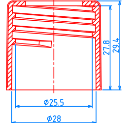
(28/水壓) CAP, P=1"x8 TPI
