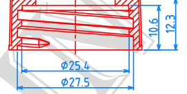
(28/400) CAP, P=1"x8 TPI
