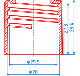
(28/水壓) CAP, P=1"x8 TPI
