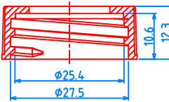
(28/400) CAP, P=1"x8 TPI
