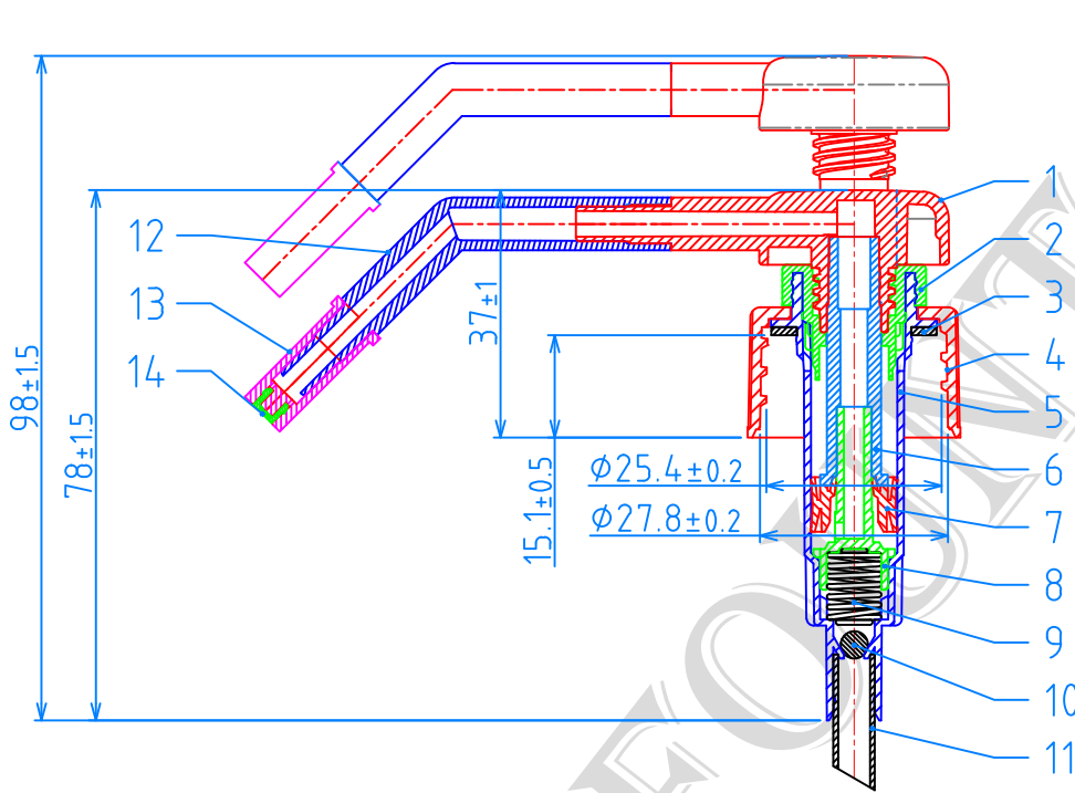
(24/400) CAP, P=1"x8 TPI
