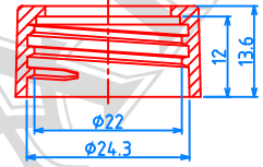
(24/410) CAP, P=1"x8 TPI
