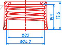
(24/415) CAP, P=1"x8 TPI
