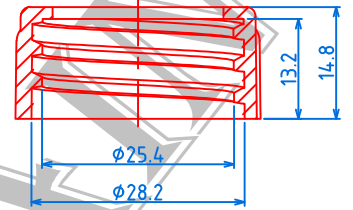
(28/400) CAP , P=1"x6 TPI
