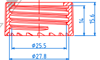
(28/400) CAP , P=1"x8 TPI
