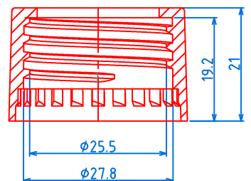
(28/410TR) CAP , P=1"x8 TPI
