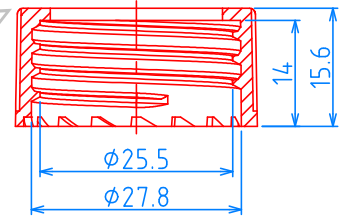
(28/400) CAP ,P=1"x8TPI
