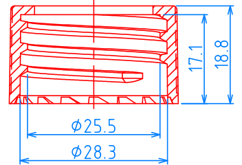
(28/410) CAP ,P=1"x6TPI
