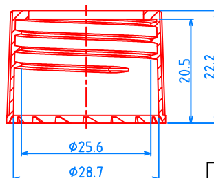
(28/400W) CAP , P=1"x8 TPI
