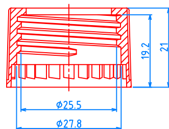
(28/410TR) CAP , P=1"x8 TPI
