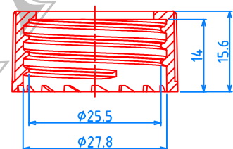
(28/400) CAP , P=1"x8 TPI
