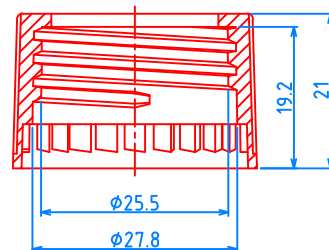
(28/410TR) CAP , P=1"x8 TPI
