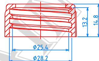
(28/400) CAP , P=1"x6 TPI
