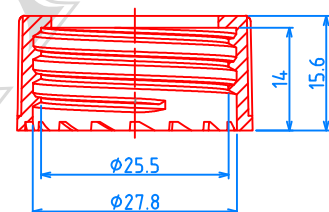
(28/400) CAP , P=1"x8 TPI
